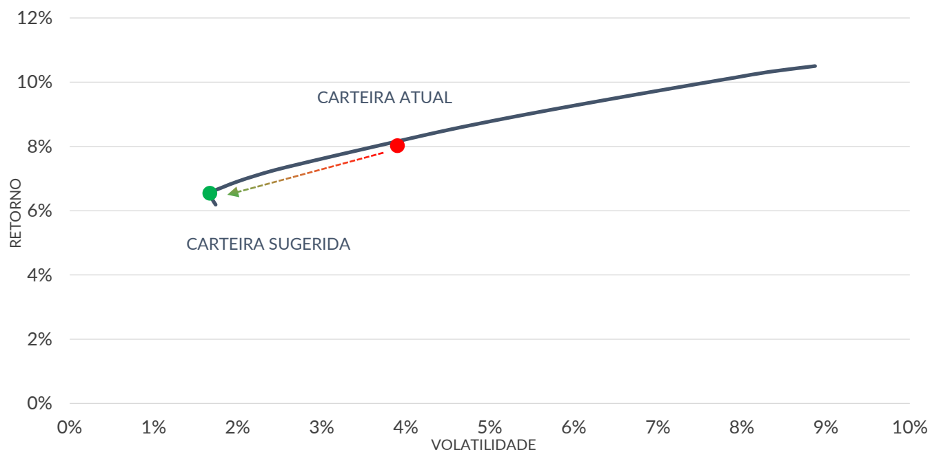
Figura 3 - Fronteira eficiente de Markowitz
